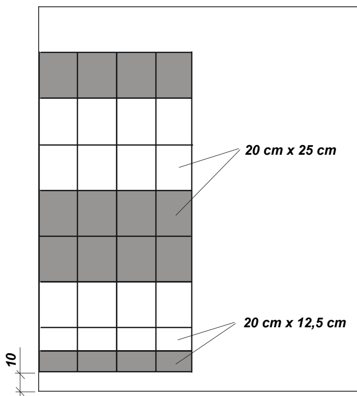
Rys. 1 Wzór okładziny ściiennej.
